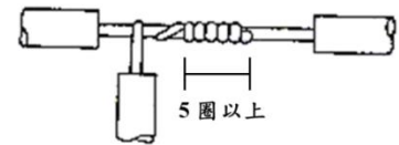
圖一五~五 實心線分歧連接法
