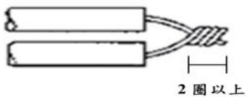
圖一五~九 實心線終端連接法
