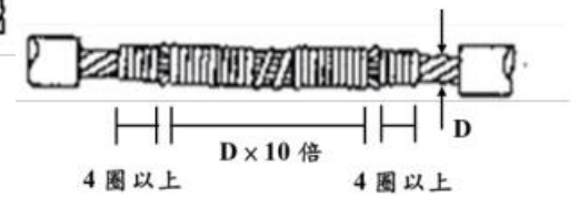
圖一五~四 絞線加紮線之延長連接法
