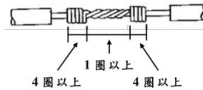
圖一五~二 實心線直接連接法
