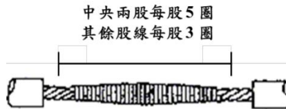
圖一五~三 絞線直接連接法
